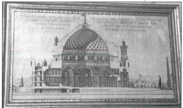
Żmien ir-Rotunda: Pjanta tar-Rotunda ddisinjata mill-arkitett G. Grognet li tinsab fis-sagrestija tal-knisja msemmija.
